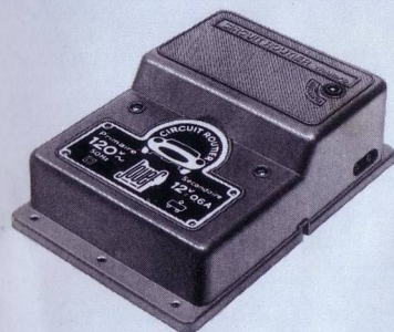
Réf. 389. TRANSFO CIRCUIT ROUTIER 600 mA Se branche sur courant alternatif. Fournit du courant continu 12 V - 0,6 A.
