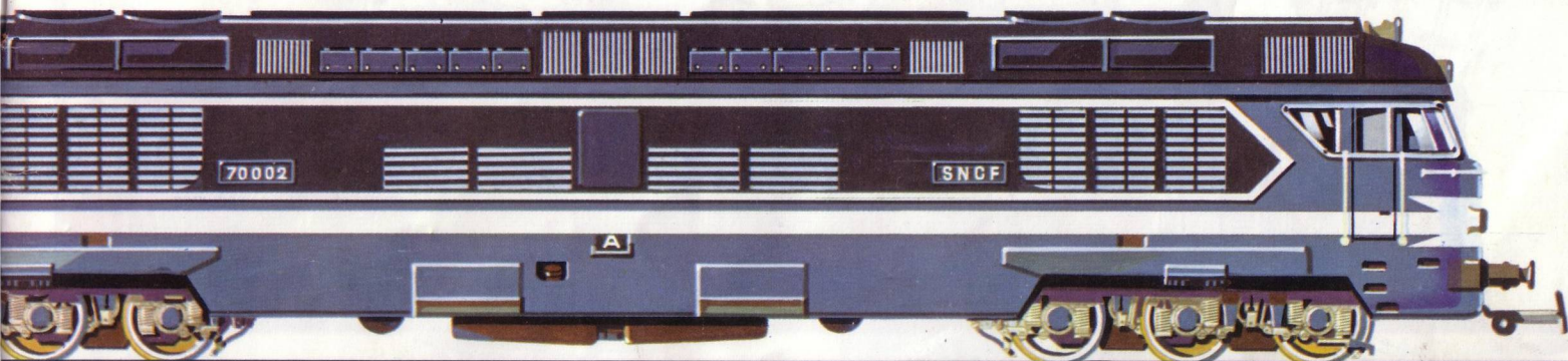
Réf. 856 E DIESEL ÉLECTRIQUE CC 70002 - Longueur 243 mm - 4 roues motrices bandagées caoutchouc.
